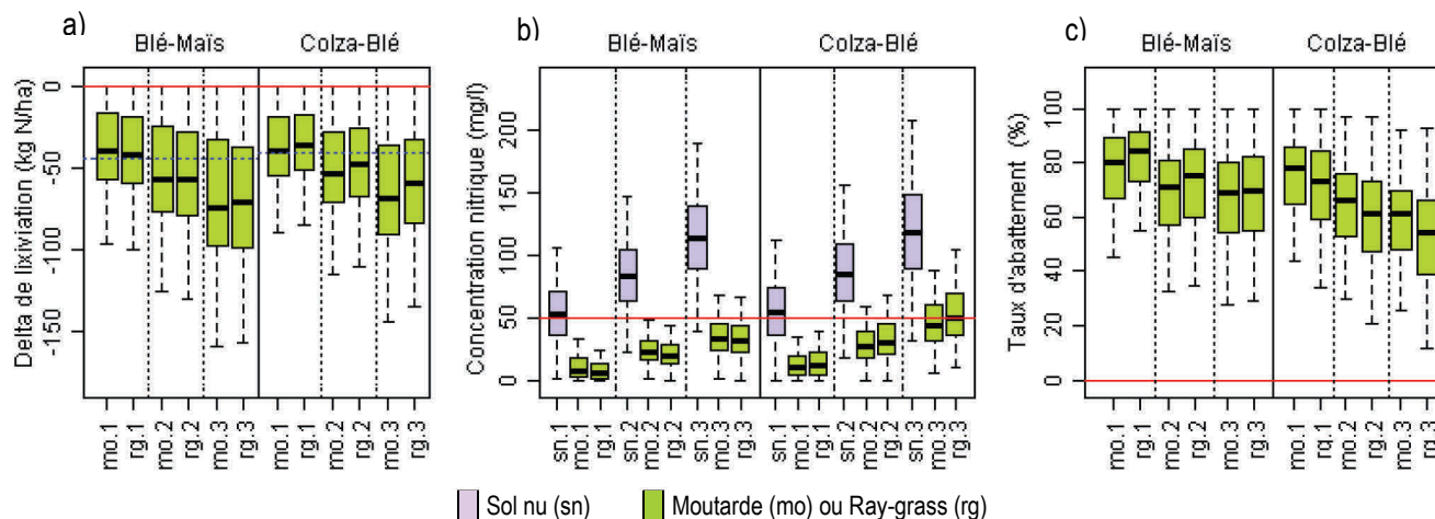
Figure 17. Effets de différentes espèces de CI sur la lixiviation de nitrate pour deux types de succession de culture Différentiel (ou delta) de lixiviation d'azote nitrique (a), concentration nitrique (b) et taux d'abattement de la concentration (c) par type de couverts, selon l'état initial en azote minéral du sol (1=20, 2=60, 3=100 kgN/ha) et la succession de culture (trait bleu = moyenne par succession) [Simulations sur tous les sites ; pour des levées aux 25/7 et 10/8, et des destructions aux 1/10 et 20/10 pour la succession colza-blé et aux 10/11 et 10/2 pour la succession blé-maïs]
