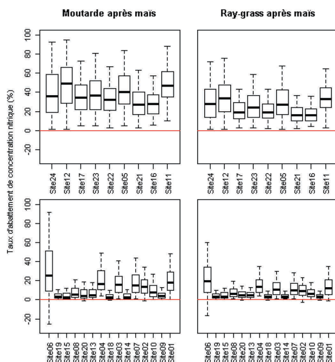
Figure 20. Taux d'abattement de la concentration nitrique avec les cultures intermédiaires (moutarde et ray-grass) en fonction des sites dans la succession maïs-maïs, fourrage (en haut) et grain (en bas)
