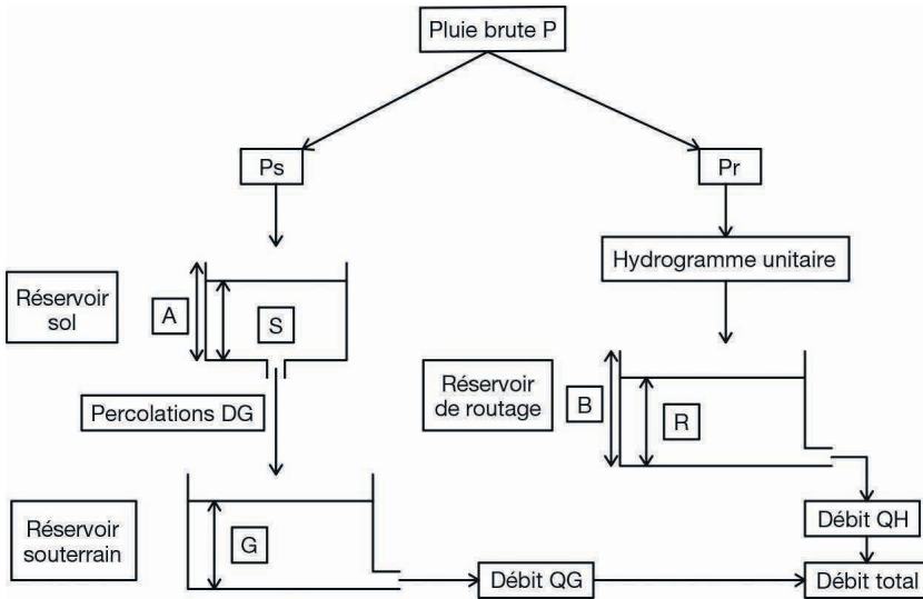
Figure 11.1. Exemple et structure d'un modèle global : le modèle GR5J (d'après Perrin, 2000). GR5J est un modèle du Génie rural à 5 paramètres journaliers. C'est un modèle global utilisé pour la simulation du débit total à l'exutoire d'un bassin versant. À partir de la pluie (P), le modèle GR5J permet de simuler le débit total à l'exutoire du bassin versant. Le bassin versant est représenté sous la forme de réservoirs (sol noté A, routage noté B et souterrain). Des variables intermédiaires, comme le débit de base (QG) et le débit de ruissellement (QH) sont calculées par le modèle.
