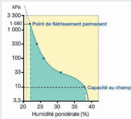
Figure 8.1. La courbe de rétention d'un sol.
